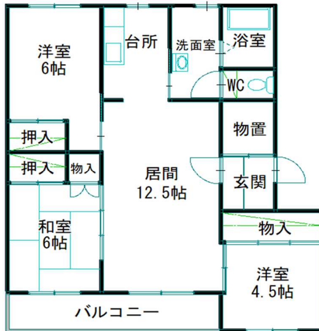
■平面図
